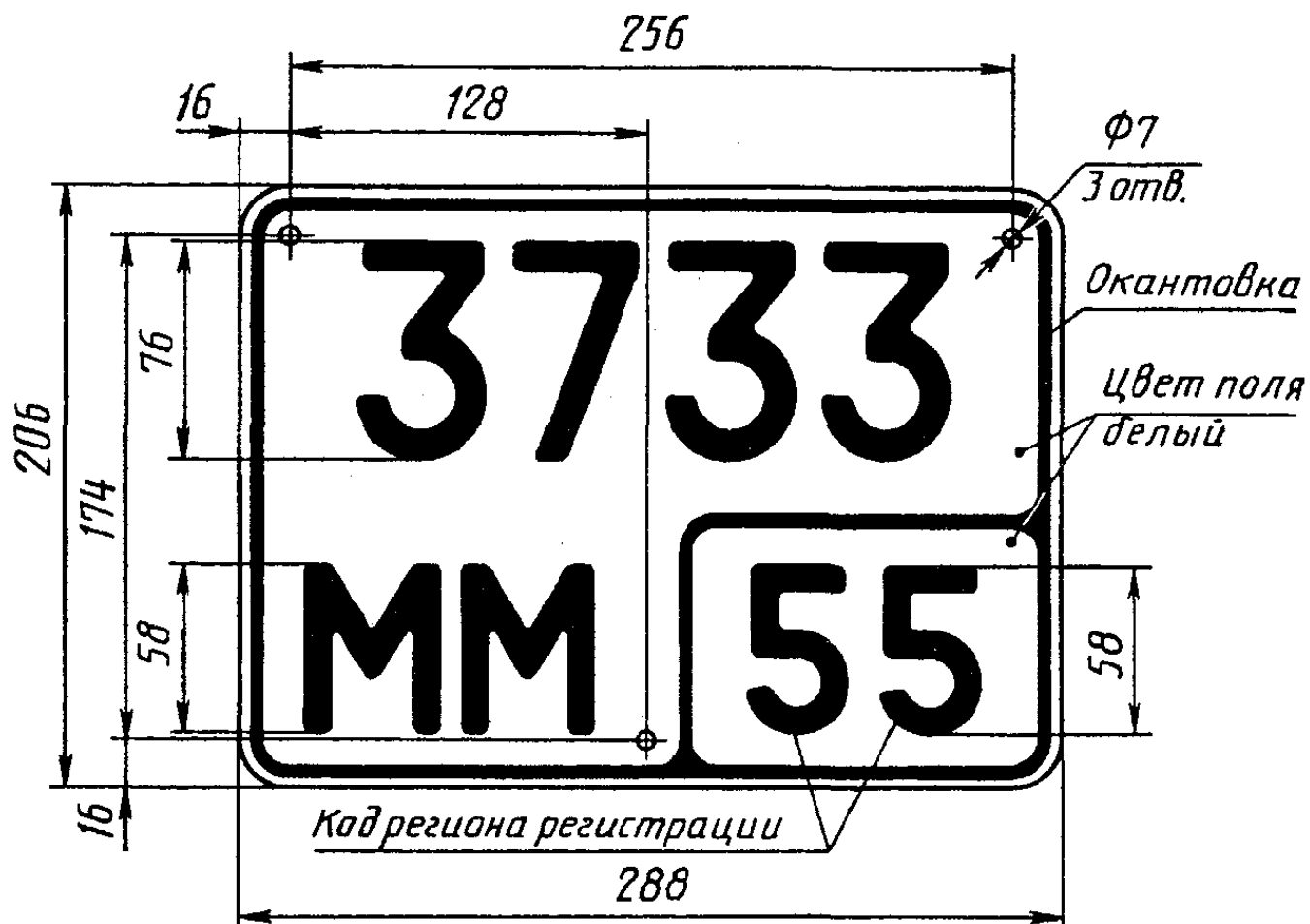
Рисунок А.6 — Регистрационный знак типа 3
