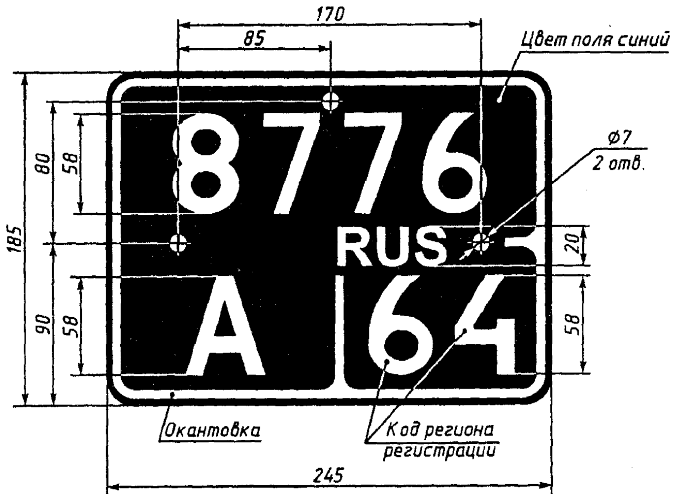
Рисунок А.22 — Регистрационный знак типа 22
