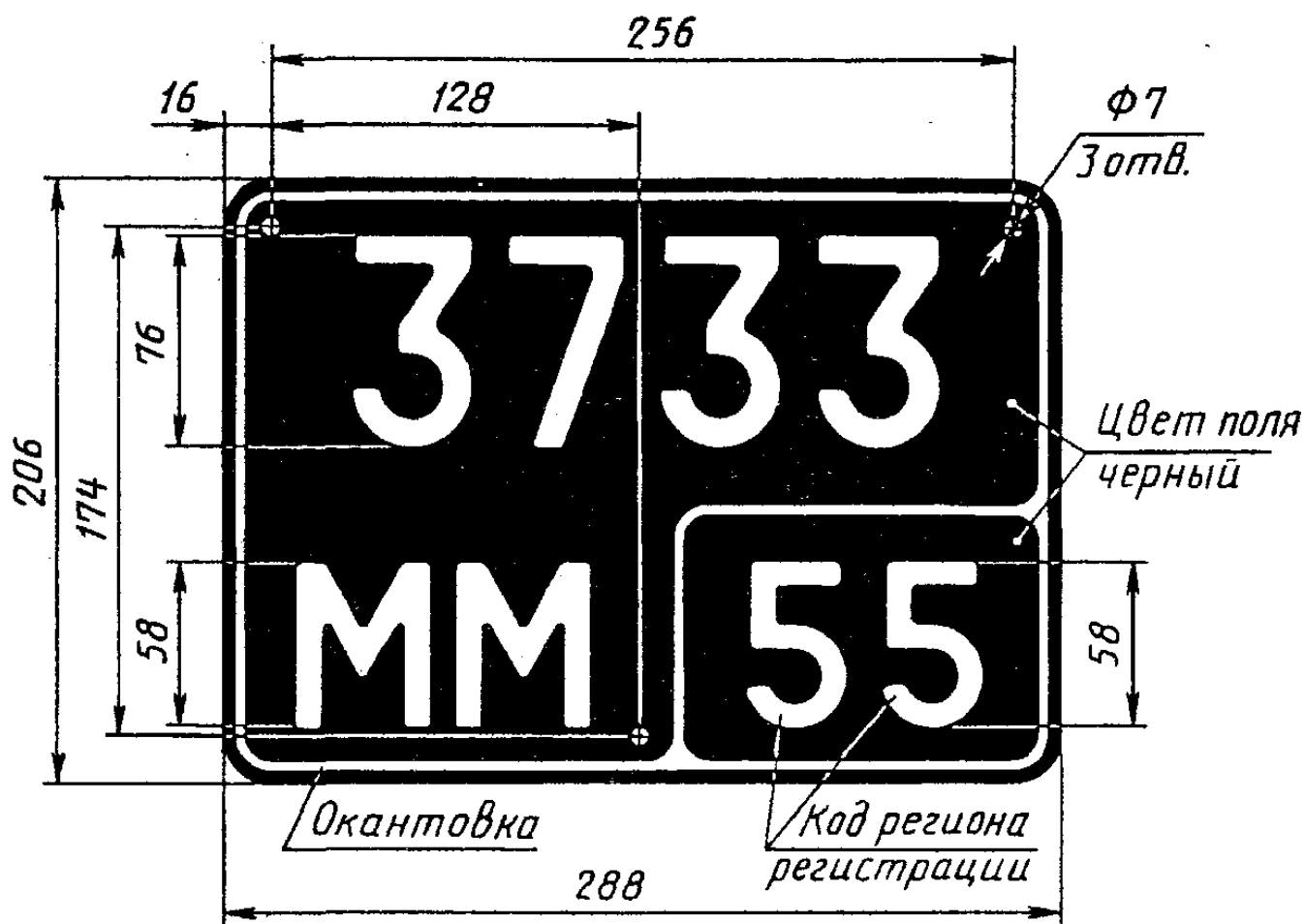
Рисунок А.10 — Регистрационный знак типа 7
