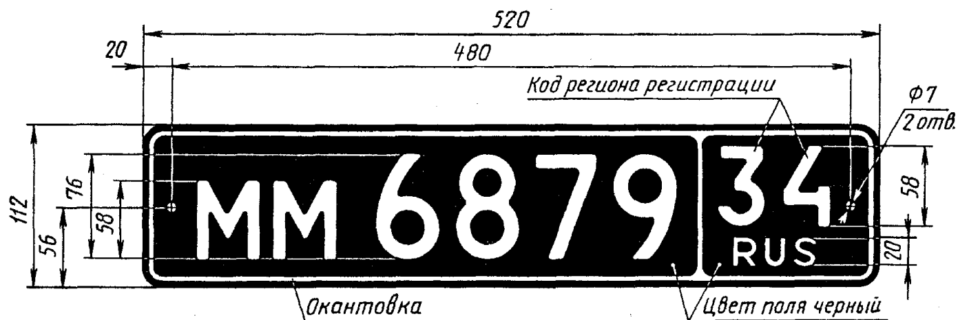
Рисунок А.9 — Регистрационный знак типа 6
