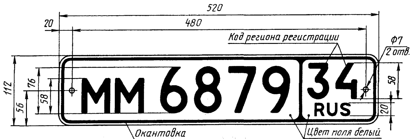
Рисунок А.5 — Регистрационный знак типа 2
